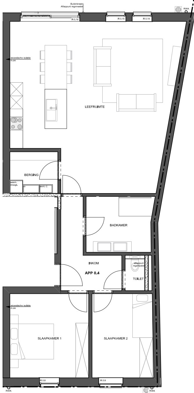
APPARTEMENT 0.4 SCHAAL: 1:100
